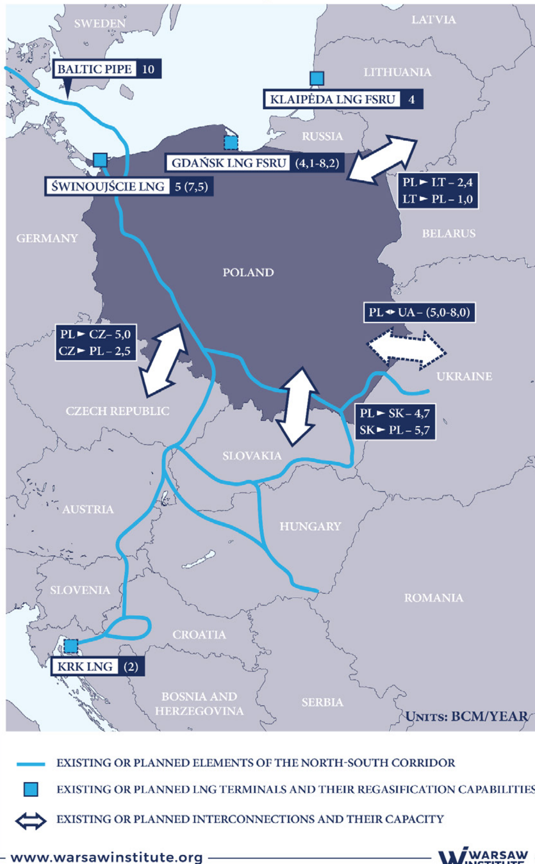
Rysunek 1. Korytarz Gazowy Północ-Południe.
